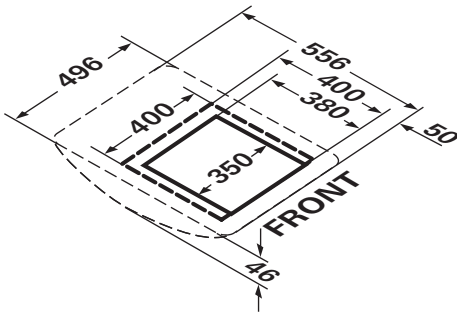
Bild 12 - Luftverteiler small
