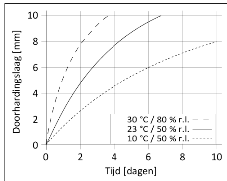
Schema 1: Uithardingsnelheid voor Sikaflex®-252
